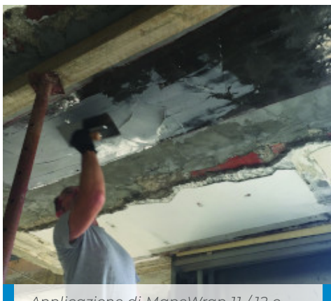
Applicazione di MapeWrap 11 / 12 o Adesilex PG1 / PG2 sul supporto
