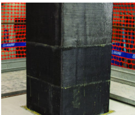
Pilastro confinato con MapeWrap C UNI-AX System
